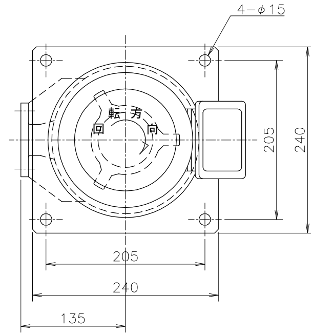
上視図
