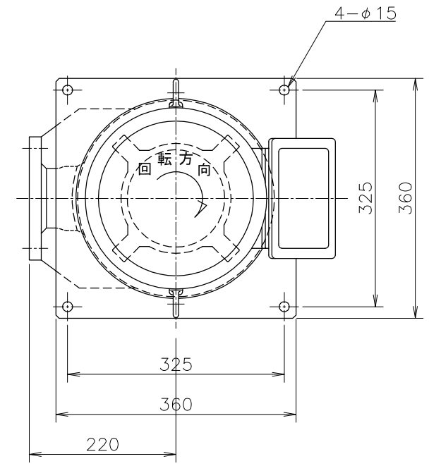
上視図
